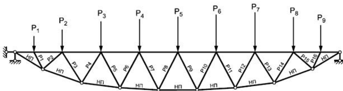
Рисунок К.1 - Расчетная схема деревометаллической фермы покрытия Крытого конькобежного центра
