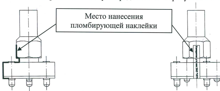
Рисунок 2.1 - Схема пломбировки от несанкционированного доступа наклономеров (вид сбоку)
